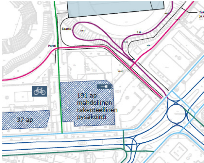
Kuva 24. Ote yleissuunnitelman reittikaaviosta alueen kaakkoisosasta.
