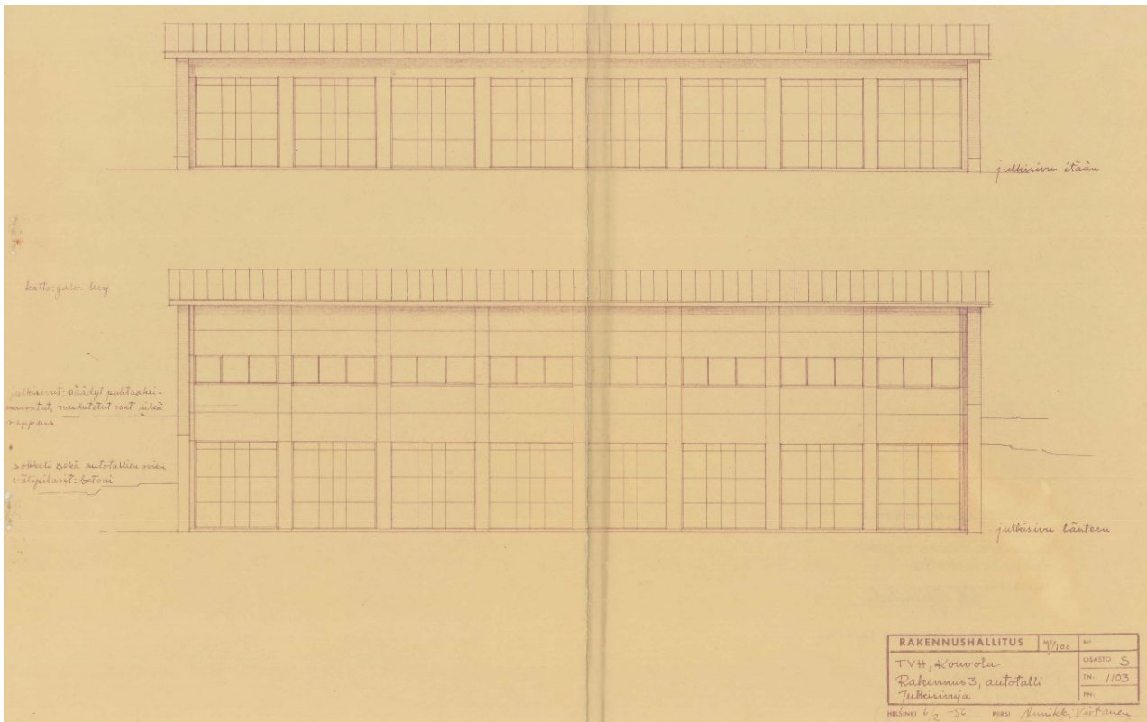
Kuva 22. TVH:n varikon rakennus 3, autotalli julkisivupiirustus. Annikki Virtanen 6.2.1956.
