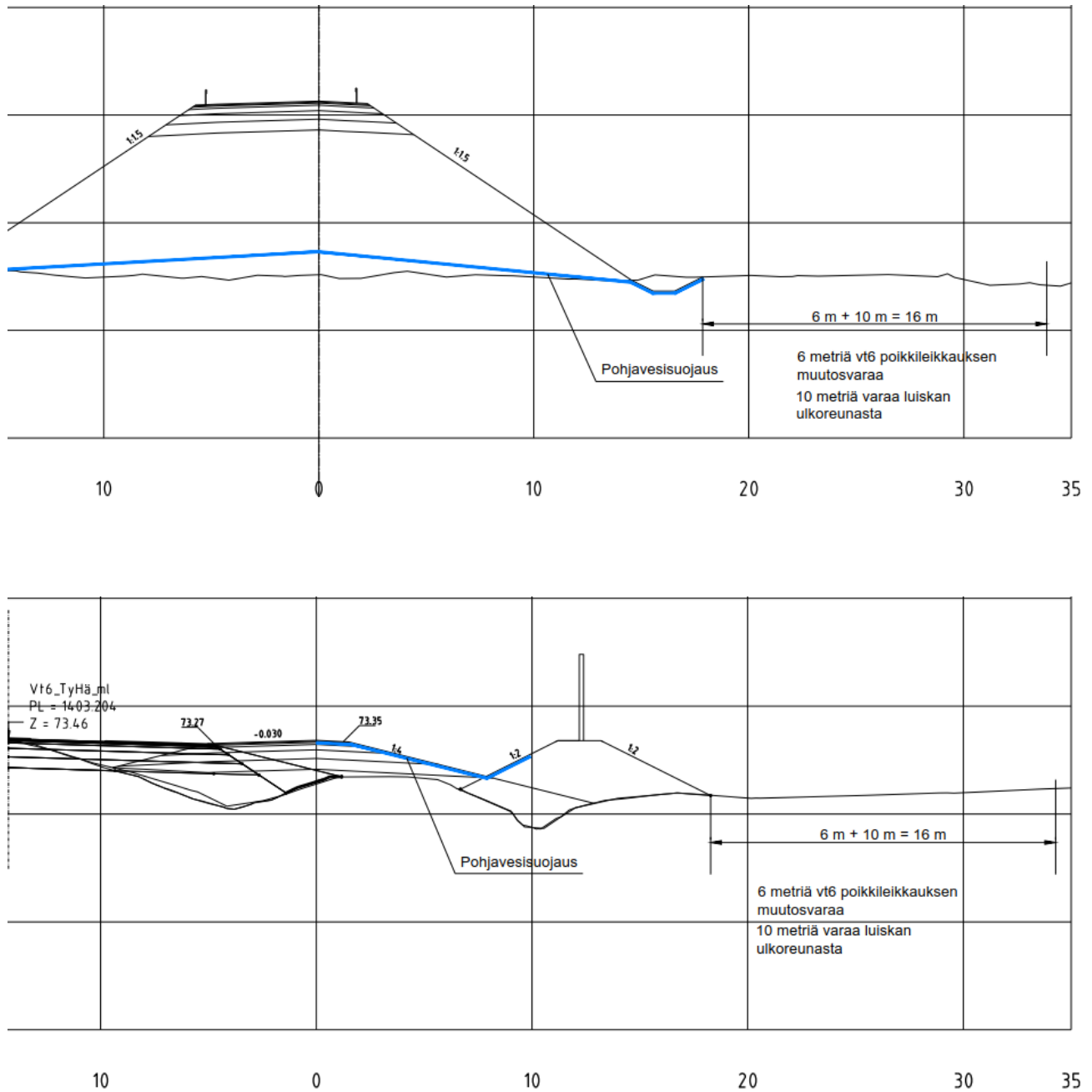
Kuva 2: Periaatepoikkileikkaukset aluevarauksen muodostumisesta
