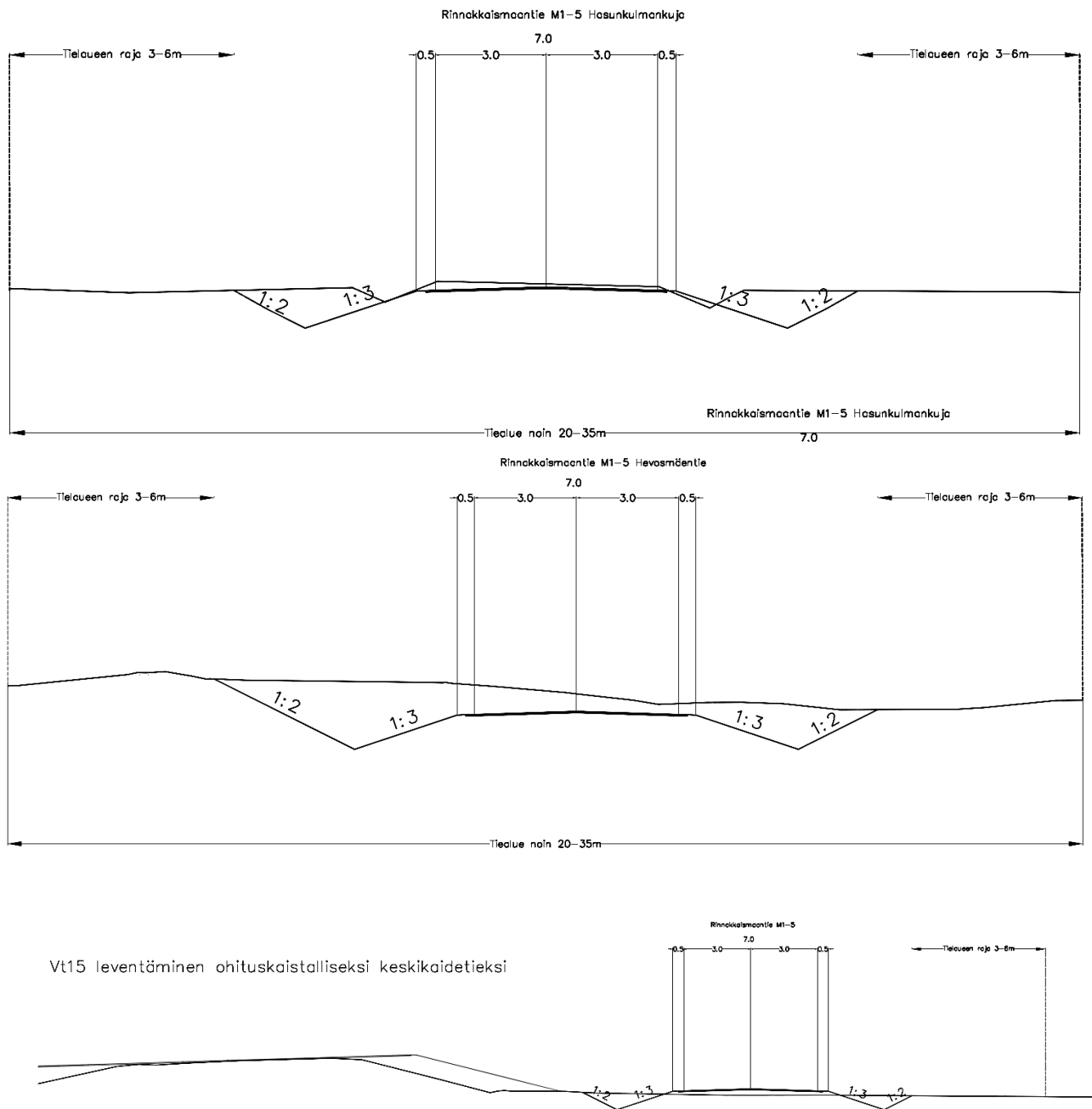
Kuva 27. Rinnakkaisteillä käytettäviä poikkileikkauksia.
