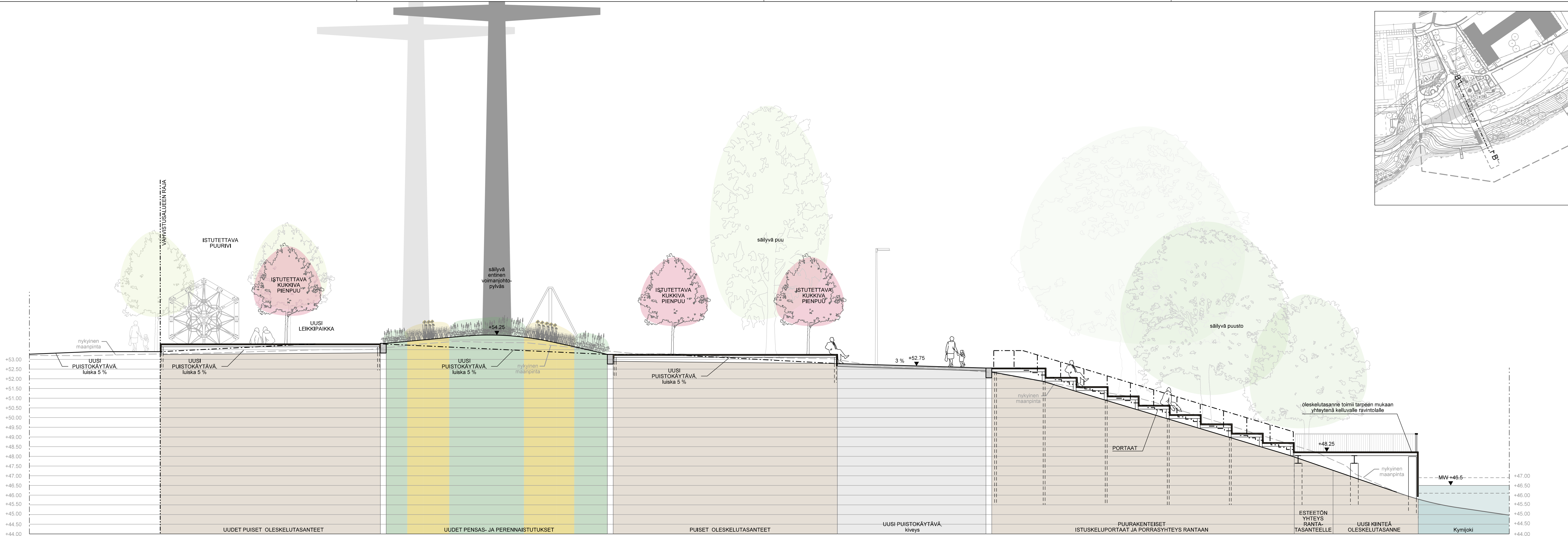
LEIKKAUS B-B', 1:100
