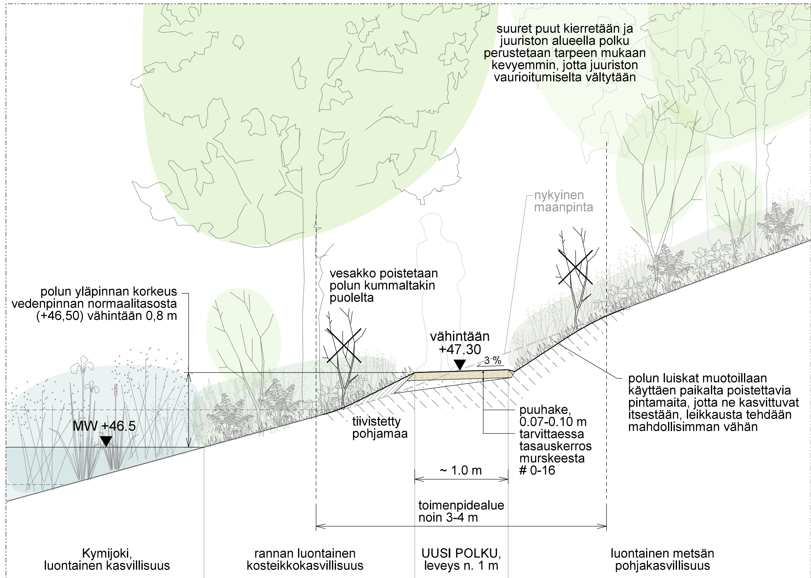
PERIAATELEIKKAUS, POLKU, 1:25
