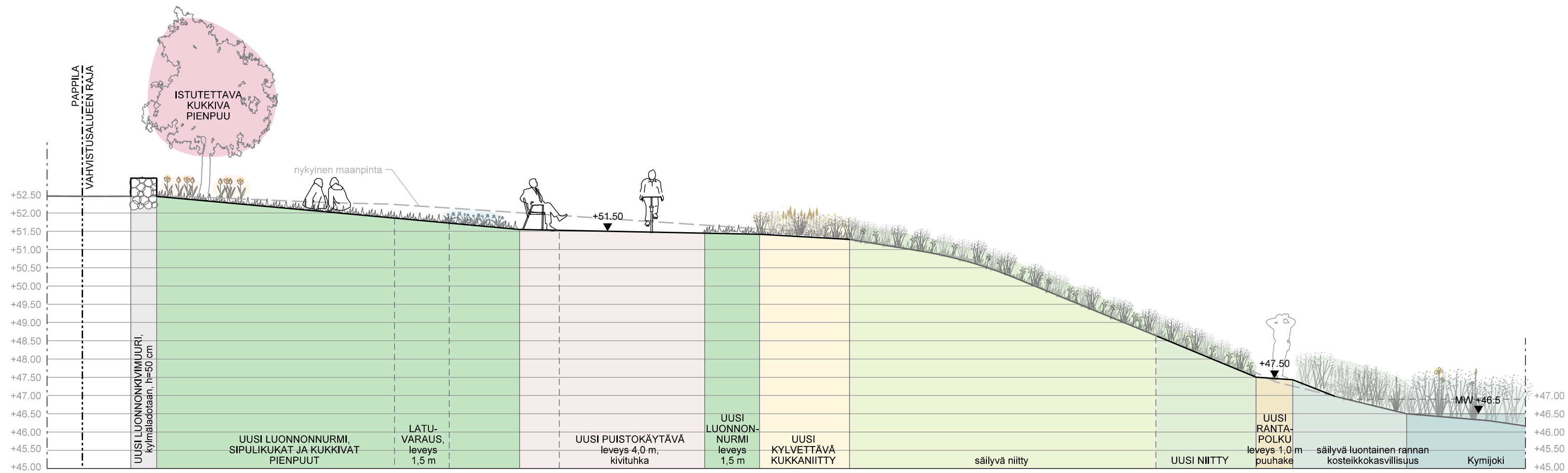
LEIKKAUS D-D', 1:100
