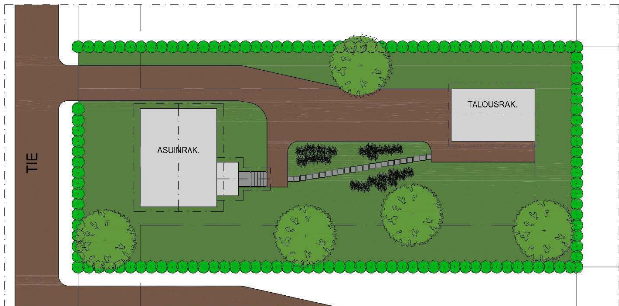
Kuva 31. Tontin pihajärjestely periaate.
