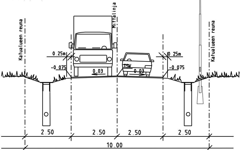
Tyypipoikkileikkaus 1:100
