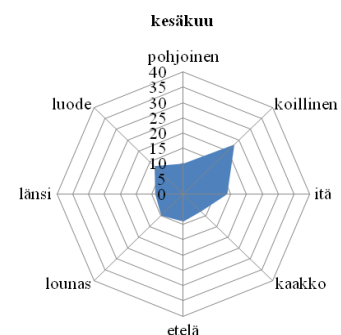
Kaavio 26. Kesäkuun tuulen suunta
