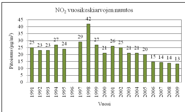
Kaavio 12. Typidioksidin (NO 2 ) vuosikeskiarvon kehitys Kouvola
