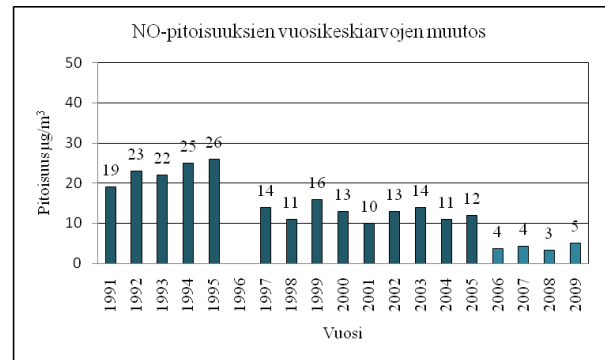
Kaavio 17. Typpimonoksidin (NO) vuosikeskiarvojen muutos
