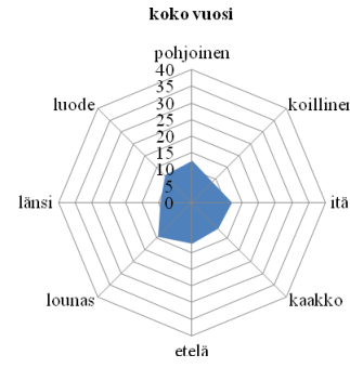
Kaavio 33. Koko vuoden tuulen suunta
