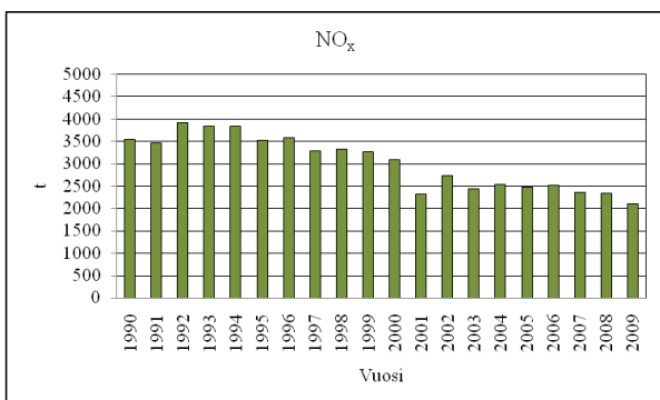
Kaavio 2. Typpioksidipäästöjen kehitys
