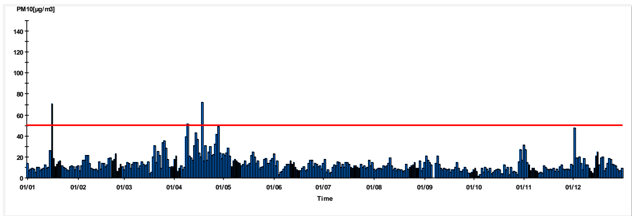
Kaavio 6. Hengitettävien hiukkasten vuorokausikeskiarvot Kouvola vuonna 2009.
