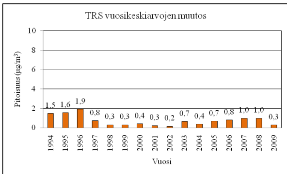
Kaavio 18. Haisevien rikkiyhdisteiden (TRS) vuosikeskiarvon muutos
