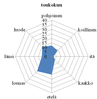
Kaavio 25. Toukokuun tuulen suunta
