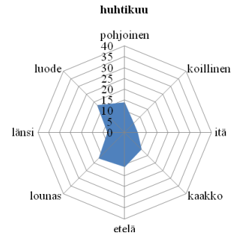
Kaavio 24. Huhtikuun tuulen suunta
