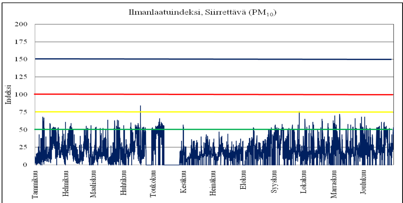
Kaavio 37. Siirrettävän aseman hengitettävien hiukkasten pitoisuus ilmanlaatuindeksinä
