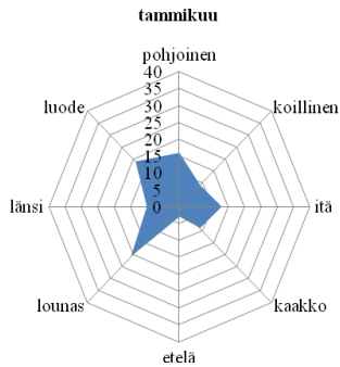
Kaavio 21. Tammikuun tuulen suunta
