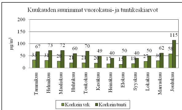
Kaavio 16. Typpidioksidin kuukauden suurimmat vuorokausi- ja tuntikeskiarvopitoisuudet
