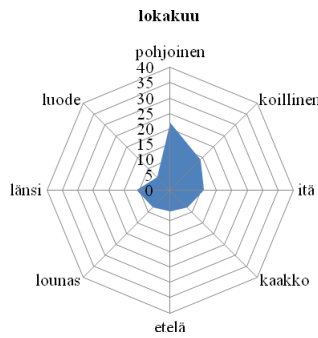
Kaavio 30. Lokakuun tuulen suunta
