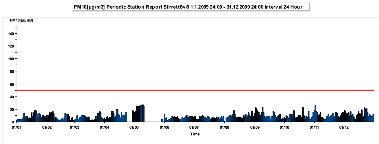
Kaavio 9. Hengitettävien hiukkasten vuorokausikeskiarvot siirrettävällä asemalla vuonna 2009.
