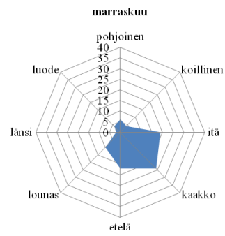
Kaavio 31. Marraskuun tuulen suunta
