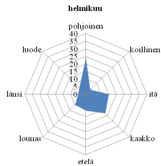
Kaavio 22. Helmikuun tuulen suunta
