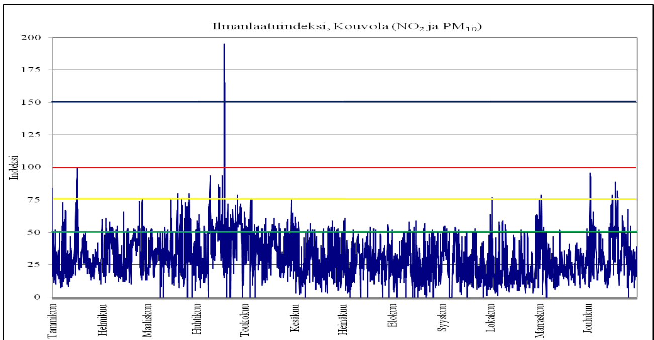
Kaavio 35. Kouvolan ilmanlaatu vuonna 2009
