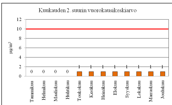
Kaavio 19. Haisevat rikkiyhdisteet (TRS) kuukauden 2. suurin vuorokausikeskiarvo ja ohjearvo 10 µg/m³
