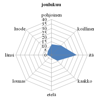
Kaavio 32. Joulukuun tuulen suunta
