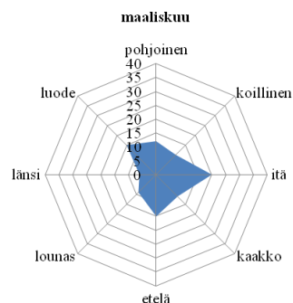
Kaavio 23. Maaliskuun tuulen suunta
