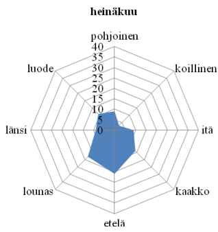
Kaavio 27. Heinäkuun tuulen suunta
