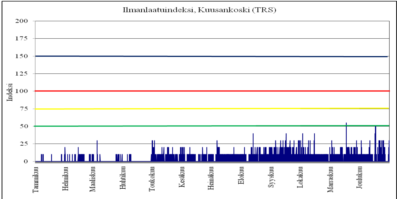
Kaavio 36. Kuusankosken TRS-pitoisuus ilmanlaatuindeksinä
