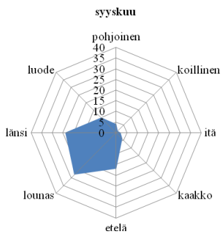
Kaavio 29. Syyskuun tuulen suunta
