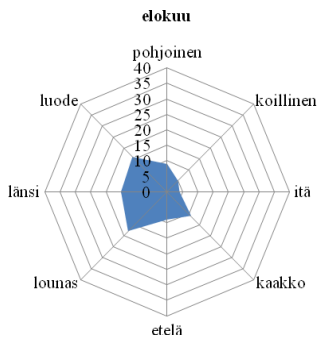
Kaavio 28. Elokuun tuulen suunta
